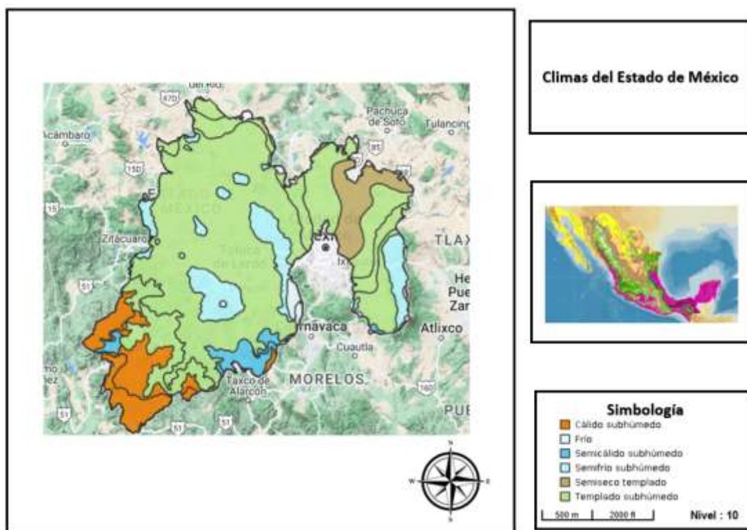
Mapa: 5. Diversidad climática del Estado de México
