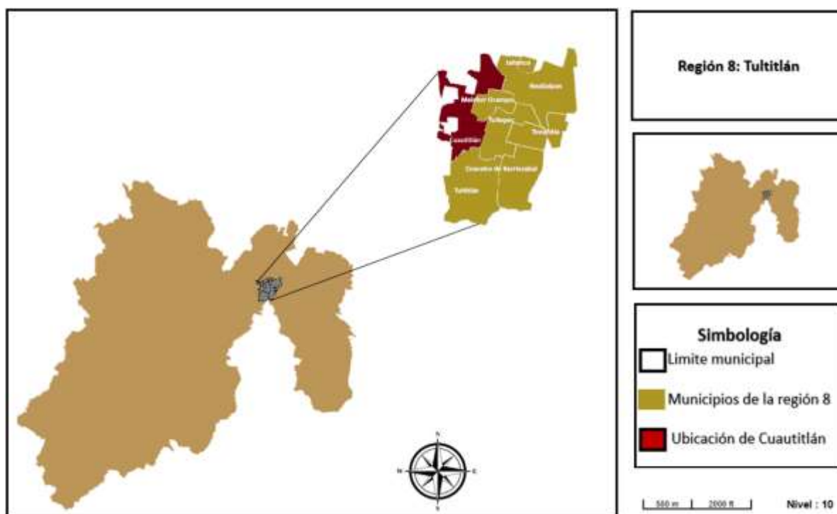
Mapa: 1. Ubicación de la región 8 del Estado de México
