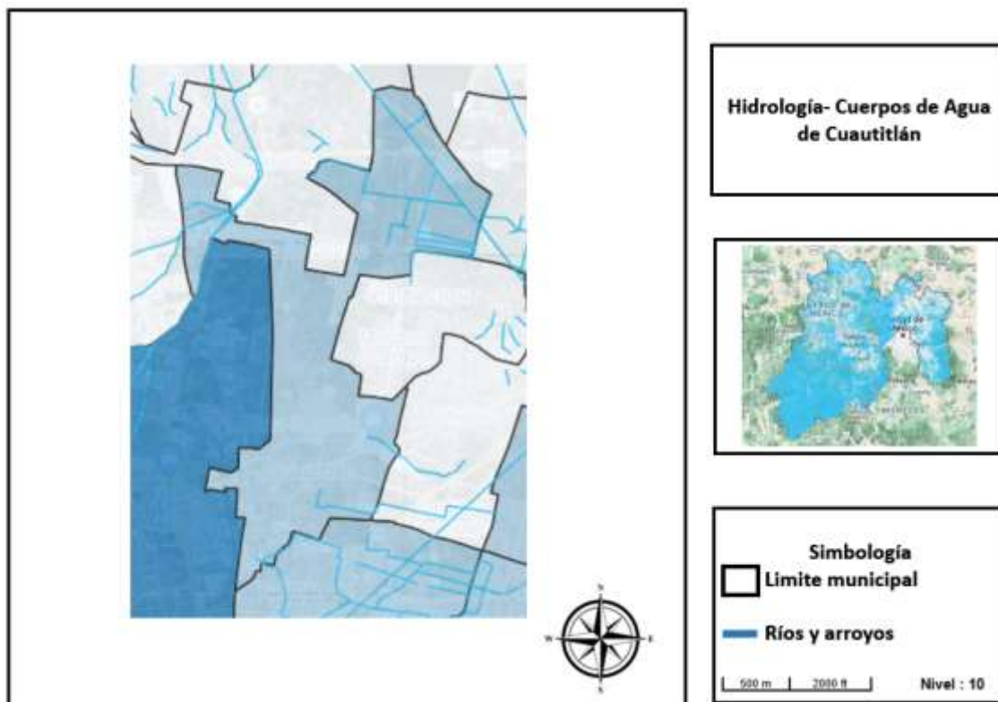
Mapa: 6. Hidrológico de Cuautitlán
