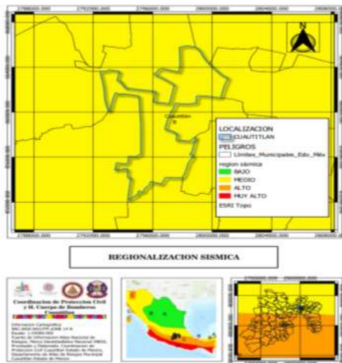
Mapa: 23. Riesgo por sismos.
